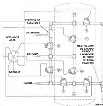
Actuador (Modelo 48-00)
