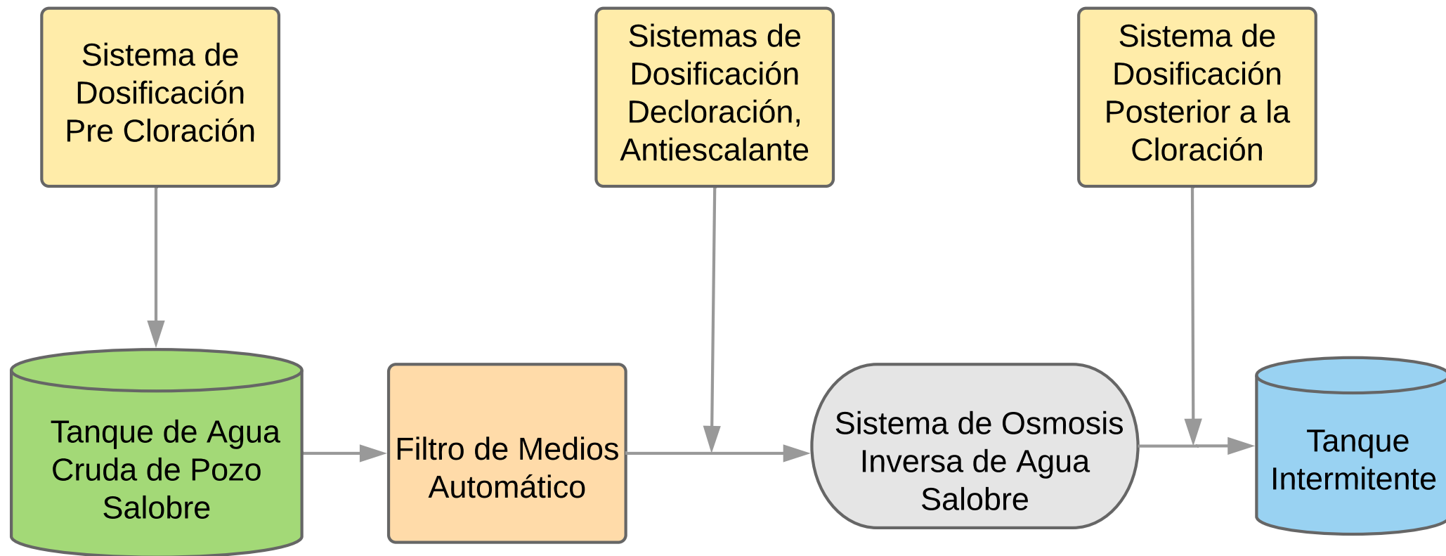
Diagrama del Sistema Industrial de Osmosis Inversa de Agua Salobre
